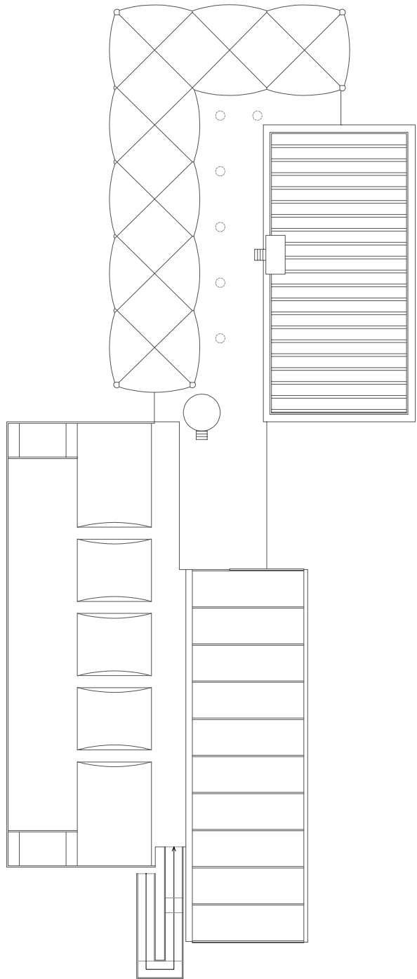
piano copertura
